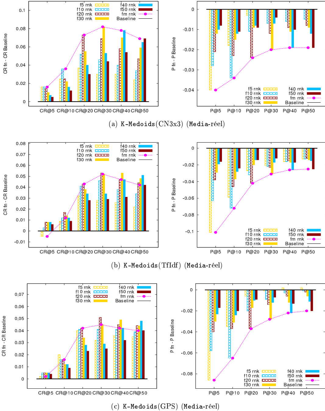
FIGURE 8.10 – Comparaison de la diff  rence entre les scores CR@m et P@m moyens de la baseline et les scores CR@m et P@m moyens de la K-Medoids avec les descripteurs (a) CN3x3, (b) Tfidf et (c) GPS sur le benchmark Media (sous-ensemble testset ) et le descripteur (d) Tree sur le benchmark Xilo en utilisant diff  rents d  coupages Fixe "fn" et une priorit   classique Rank dans un cas r  el
