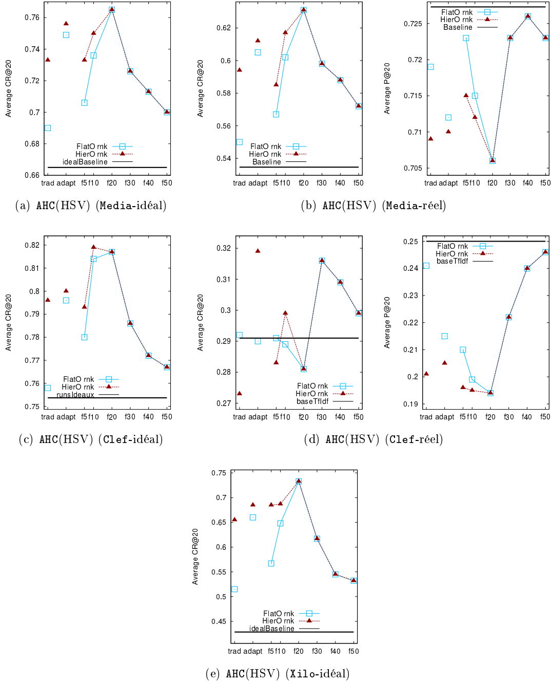
FIGURE 7.11 – Comparaison des techniques de réordonnancement sur plusieurs benchmarks pour CR@20. Les scores CR@20 et P@20 moyens représentent la AHC avec le descripteur HSV en utilisant différentes techniques de découpage (en abscisse) et une priorité classique Rank dans un cas idéal et réel sur les benchmarks (a) (b) Media (sous-ensemble testset ), (c) (d) Clef et (e) Xilo
