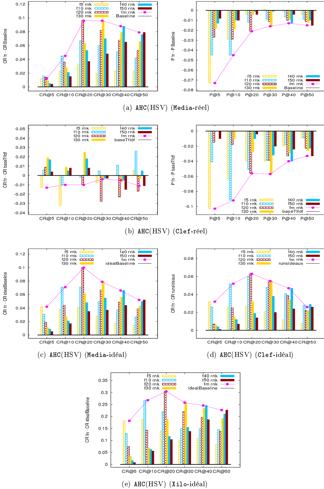
FIGURE 7.8 – Comparaison de la différence entre les scores CR@m et P@m moyens de la baseline et les scores CR@m et P@m moyens de la AHC avec HSV en utilisant différents découpages Fixe "fn" et une priorité Rank dans un cas réel et idéal sur les benchmarks (a) (c) Media (sous-ensemble testset ), (b) (d) Clef et (e) Xilo
