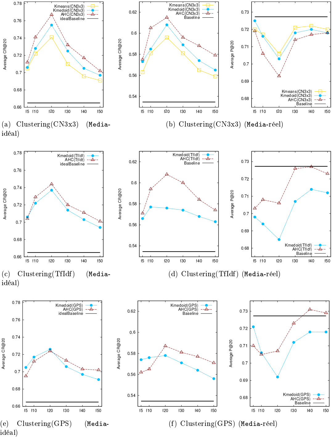
FIGURE A.7 – Comparaison des méthodes de clustering sur plusieurs descripteurs. Les scores CR@20 et P@20 moyens représentent les méthodes K-Means, K-Medoids et AHC avec les descripteurs (a) (b) CN3x3, (c) (d) TfIdf et (e) (f) GPS en utilisant différentes techniques de découpage (en abscisse) et une priorité par Rank dans un cas idéal et réel sur le benchmark Media (sous-ensemble testset)
