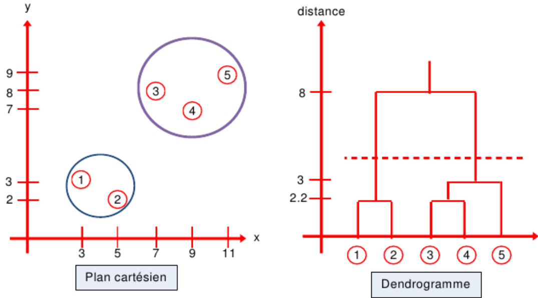
FIGURE 3.1 – (à gauche) L'ensemble de documents représentés dans un plan cartésien. (à droite) Exemple du dendrogramme ou hiérarchie de clusters généré par la AHC avec les 5 documents
