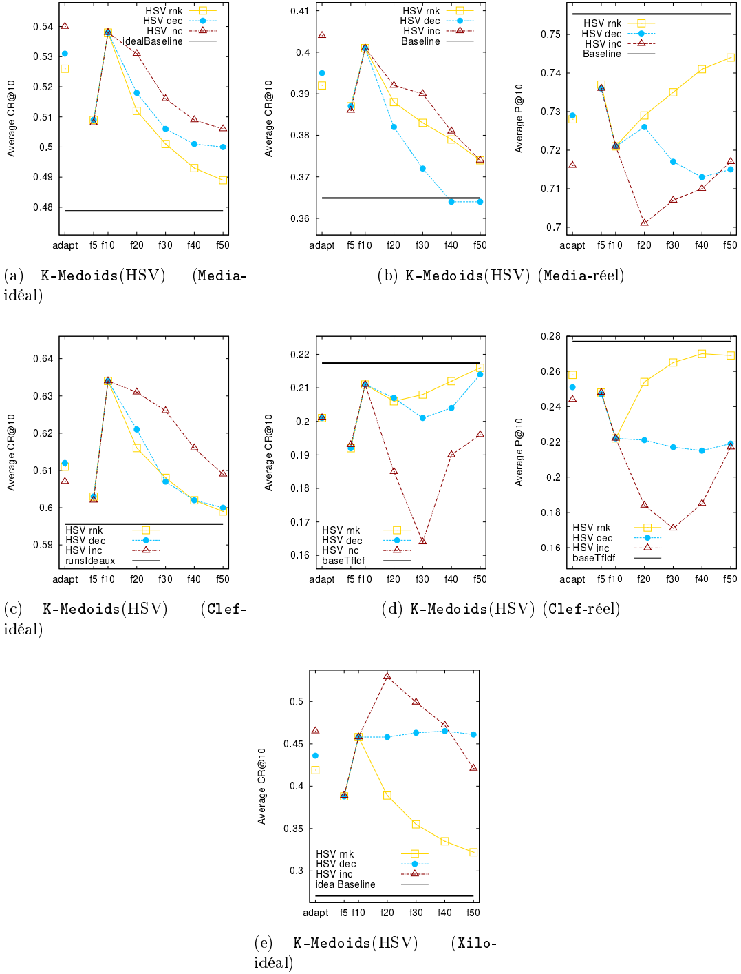
FIGURE 8.5 – Comparaison des techniques de priorité sur plusieurs benchmarks. Les scores CR@10 et P@10 moyens représentent K-Medoids avec le descripteur HSV en utilisant différentes techniques de découpage (en abscisse) dans un cas idéal et réel sur les benchmarks (a) (b) Media (sous-ensemble testset ), (c) (d) Clef et (e) Xilo
