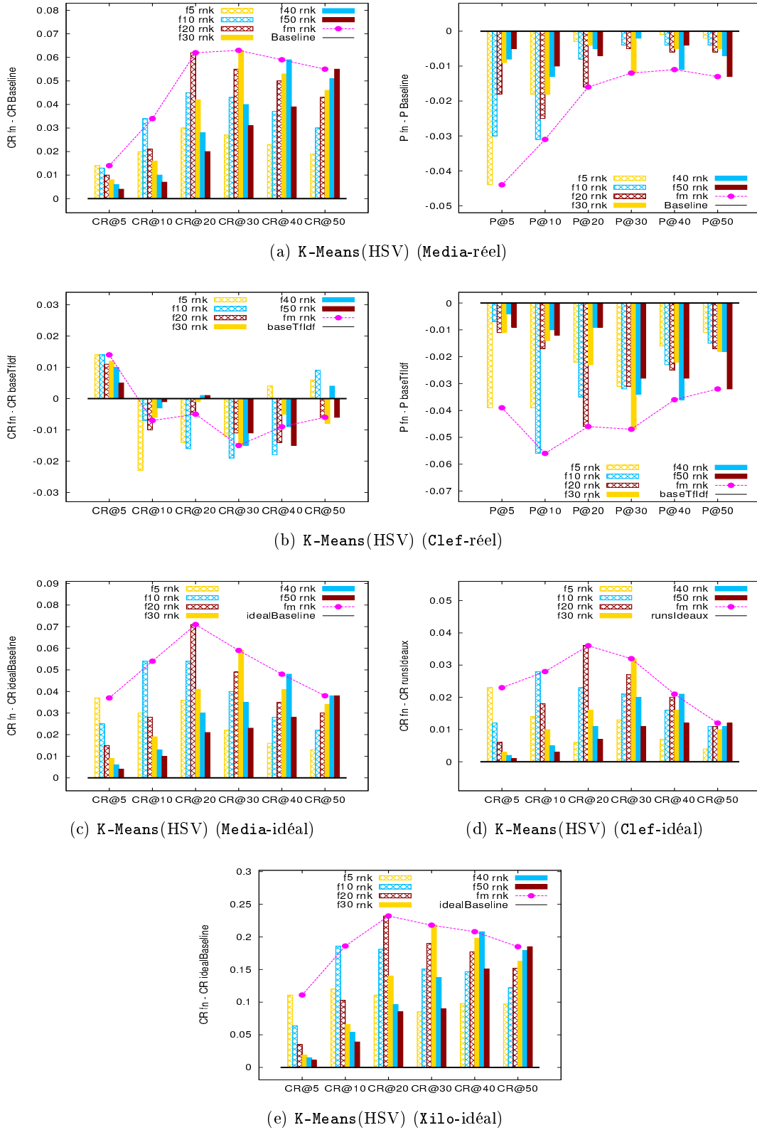
FIGURE 8.3 – Valeur maximale pour CR@m sur plusieurs benchmarks. Les scores repr  sentent la diff  rence entre les scores CR@m , P@m moyens de la baseline et les scores CR@m , P@m moyens de la K-Means avec HSV en utilisant diff  rents d  coupages "fn" et une priorit   Rank sur les benchmarks (a) (c) Media-testset, (b) (d) Clef et (e) Xilo
