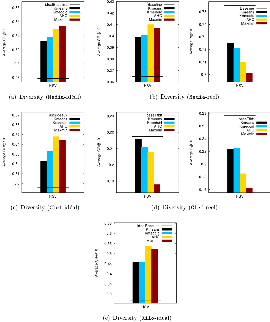
FIGURE 9.10 – Comparaison des méthodes de diversité sur plusieurs benchmarks. Les scores CR@10 et P@10 moyens représentent les méthodes K-Means, K-Medoids, AHC et Maxmin avec le descripteur HSV en utilisant les paramètres mentionnés dans le tableau 9.1 dans un cas idéal et réel sur les benchmarks (a) (b) Media (sous-ensemble testset), (c) (d) Clef et (e) Xilo
