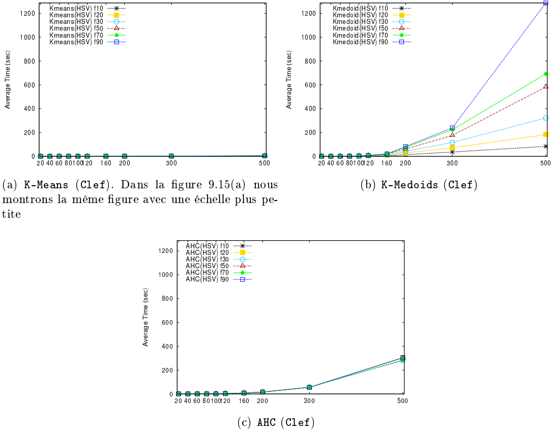
FIGURE 9.14 – Comparaison du temps de calcul des méthodes de clustering sur plusieurs nombres des clusters. Le temps de calcul représente la moyenne des 39 requêtes du benchmark Clef sur (a) K-Means , (b) K-Medoids et (c) la AHC avec le descripteur HSV en utilisant différents nombres d’images (en abscisse)
