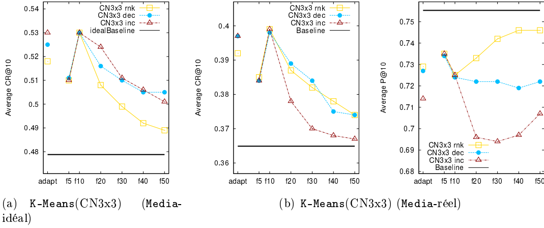
FIGURE 8.2 – Comparaison des techniques de priorité sur le descripteur CN3x3. Les scores CR@10 et P@10 moyens représentent la méthode K-Means avec le descripteur CN3x3 en utilisant différentes techniques de découpage (en abscisse) dans un cas idéal et réel sur le benchmark Media (sous-ensemble testset)
