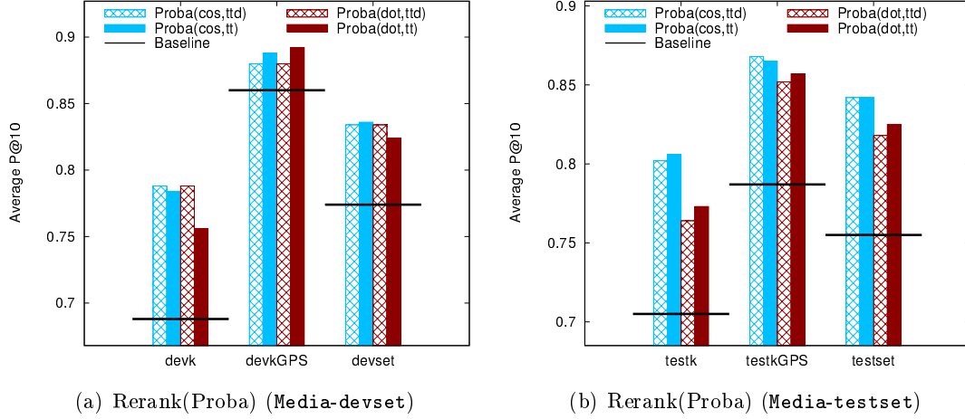
FIGURE 6.14 – Comparaison des descripteurs Proba(cos) vs Proba(dot). Les scores P@10 moyens représentent le Rerank avec le descripteur "Proba" en utilisant les mesures de similarité "cos" (en bleu) et "dot" (en rouge) avec différents champs de métadonnées (tt, ttd) dans un cas réel sur le benchmark Media (a) sous-ensemble devset et (b) sous-ensemble testset
