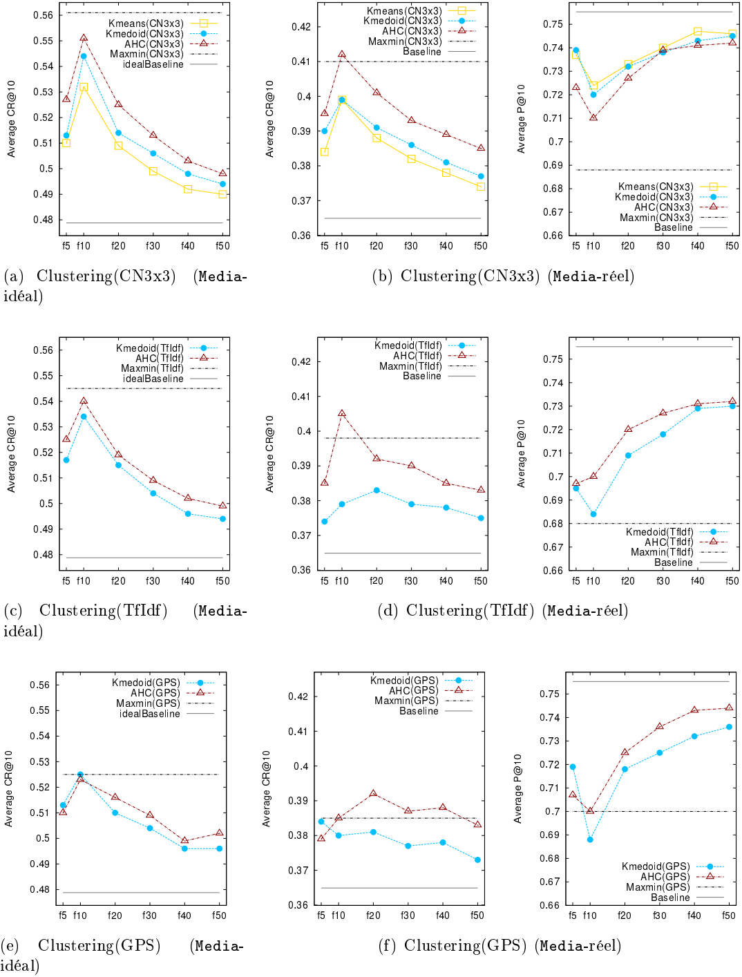
FIGURE 9.4 – Comparaison des méthodes de clustering sur plusieurs descripteurs. Les scores CR@10 et P@10 moyens représentent les méthodes K-Means, K-Medoids, AHC et Maxmin avec les descripteurs (a) (b) CN3x3, (c) (d) TfIdf et (e) (f) GPS en utilisant différentes techniques de découpage (en abscisse) et une priorité par Rank dans un cas idéal et réel sur le benchmark Media (sous-ensemble testset )
