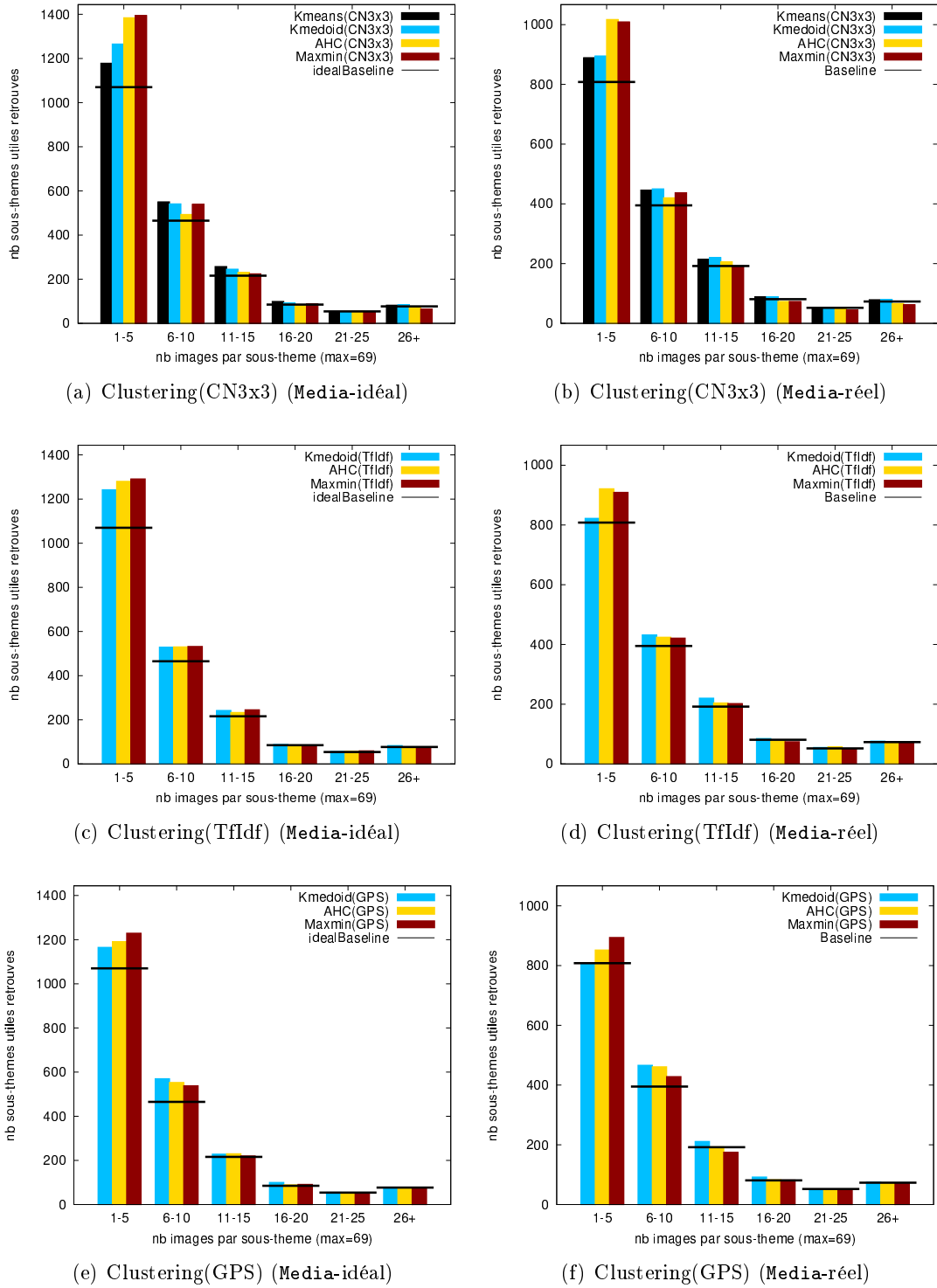
FIGURE 9.9 – Apport des sous-thèmes utiles retrouvés dans les 10 premiers résultats des méthodes K-Means, K-Medoids, AHC et Maxmin avec les descripteurs (a) (b) CN3x3, (c) (d) TfIdf et (e) (f) GPS en utilisant un découpage Fixe à 10 clusters et une priorité par Rank dans un cas idéal et réel sur le benchmark Media (sous-ensemble testset )
