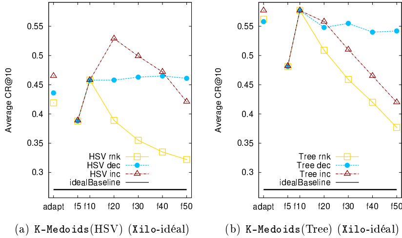
FIGURE 8.6 – Comparaison des techniques de priorité avec les descripteurs HSV et Tree. Les scores CR@10 et P@10 moyens représentent K-Medoids avec les descripteurs (a) HSV et (b) Tree en utilisant différentes techniques de découpage (en abscisse) dans un cas idéal sur le benchmark Xilo
