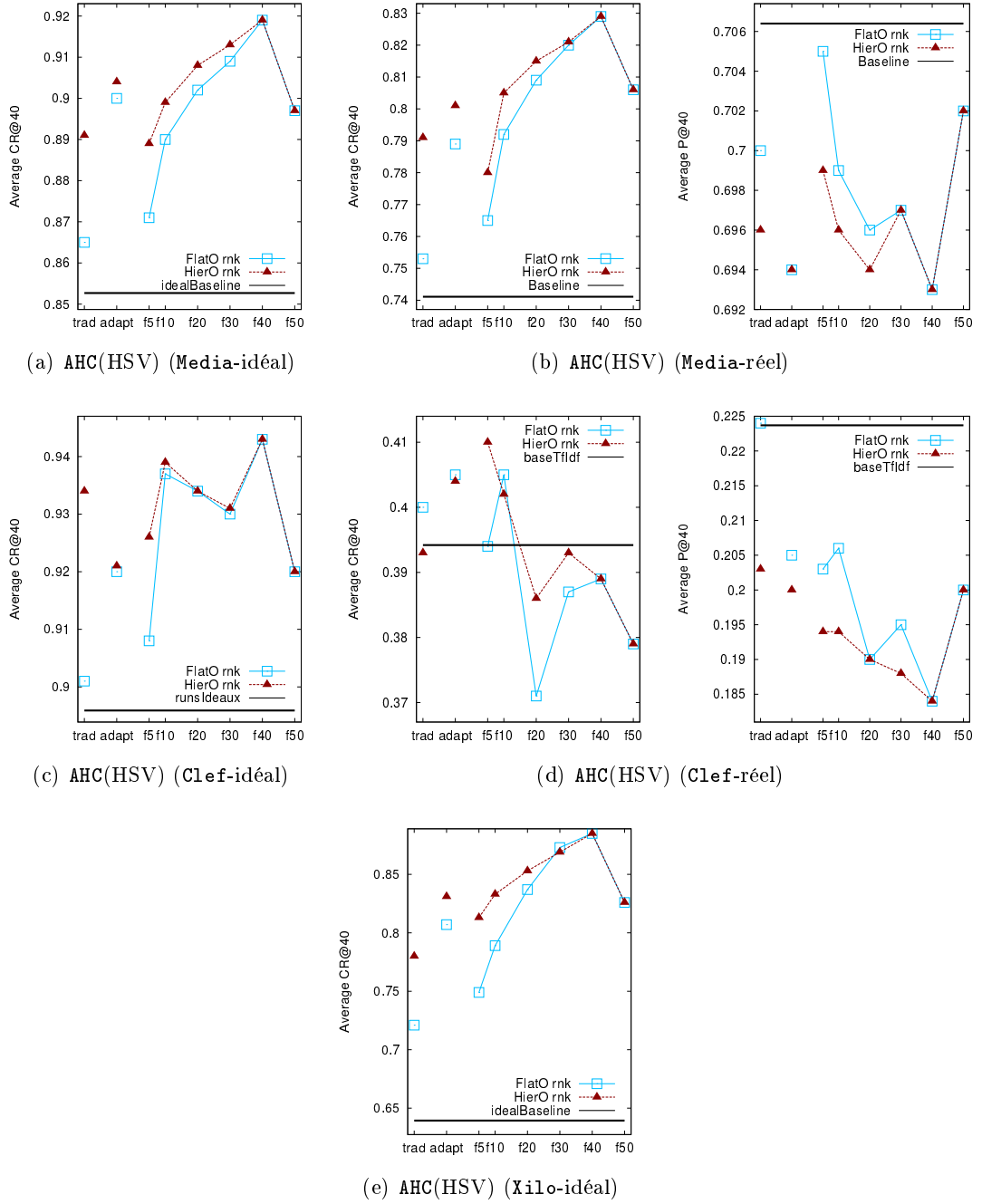
FIGURE A.4 – Comparaison des techniques de réordonnancement sur plusieurs benchmarks pour CR@40. Les scores CR@40 et P@40 moyens représentent la AHC avec le descripteur HSV en utilisant différentes techniques de découpage (en abscisse) et une priorité classique Rank dans un cas idéal et réel sur les benchmarks (a) (b) Media (sous-ensemble testset ), (c) (d) Clef et (e) Xilo
