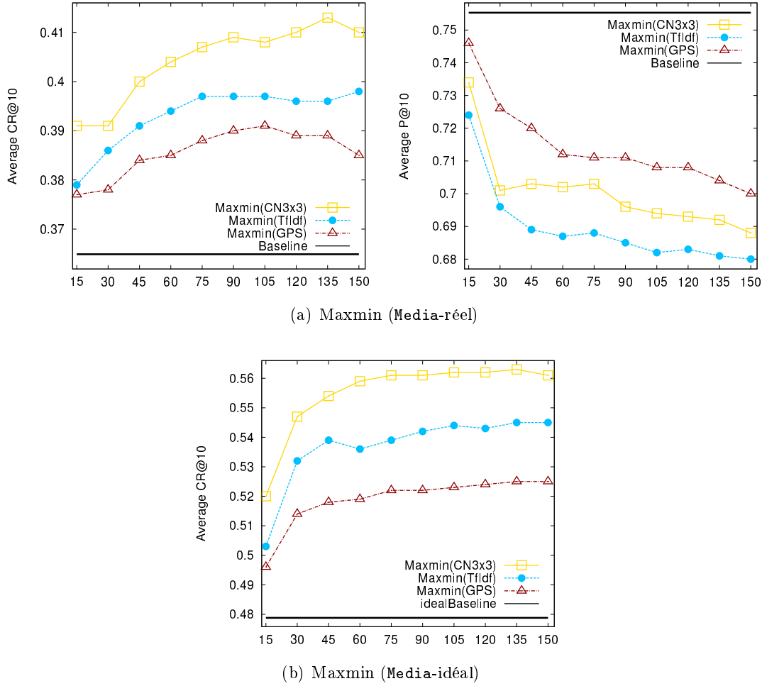
FIGURE 9.2 – Comparaison de Maxmin avec différents nombres d’images (en abscisse) sur plusieurs descripteurs. Les scores CR@10 et P@10 moyens représentent Maxmin avec les descripteurs CN3x3, Tfidf et GPS dans un cas idéal et réel sur le benchmark Media (sous-ensemble testset )
