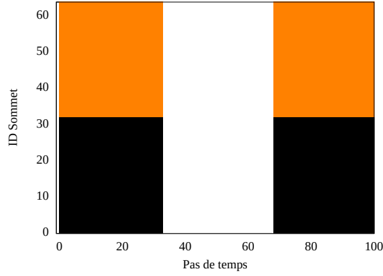
FIGURE 6.4 – Vérité terrain du motif merge-split (pas de temps en abscisse, identifiant sommet en ordonnée)
