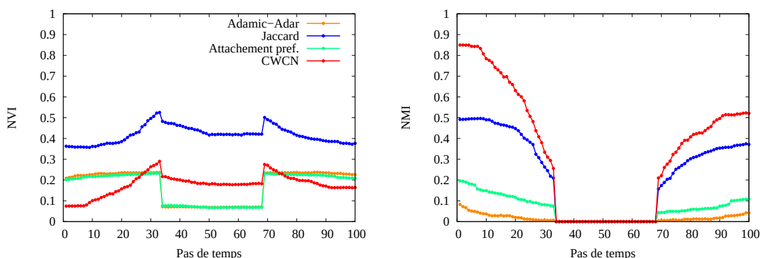
FIGURE 6.5 – Comparaison des mesures de préférences pour merge-split (100 pas de temps) : à gauche NVI (à minimiser), à droite NMI (à maximiser)
